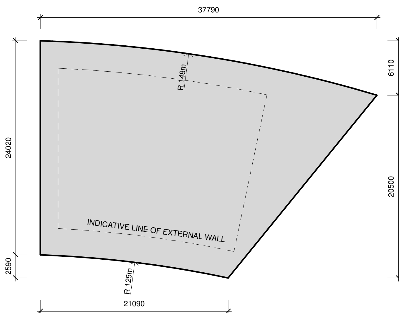
1 Low Level Plan DA3-009 1 : 250
